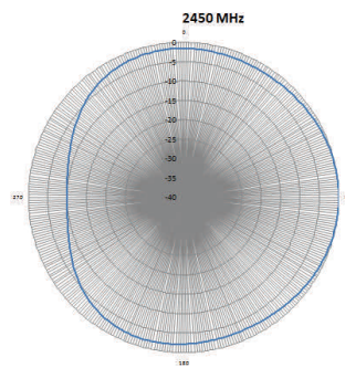
H-Plane Pattern
